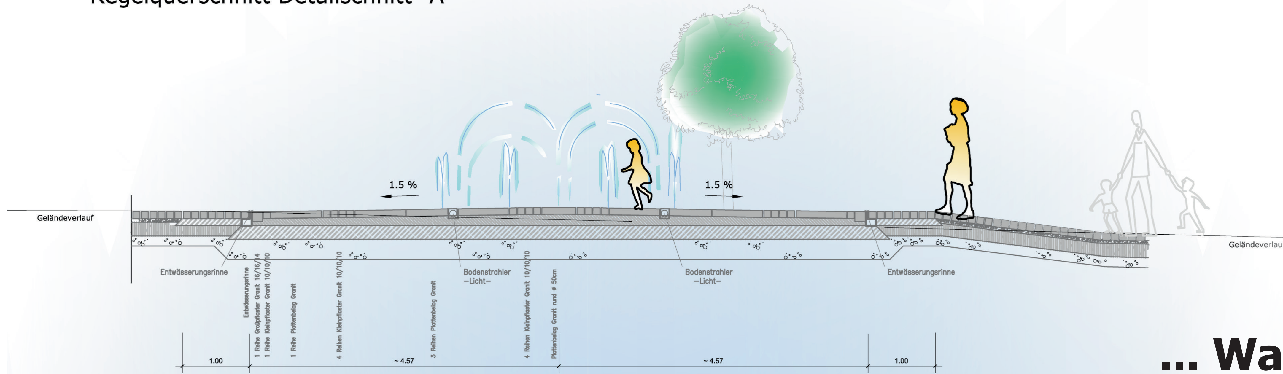
Detail "1" Regelquerschnitt Detailschnitt "A"
